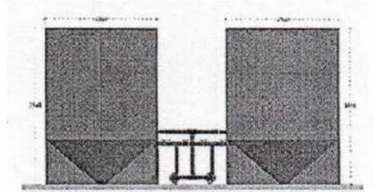
Ilustración 1. Esquema del tanque de preclarificación
